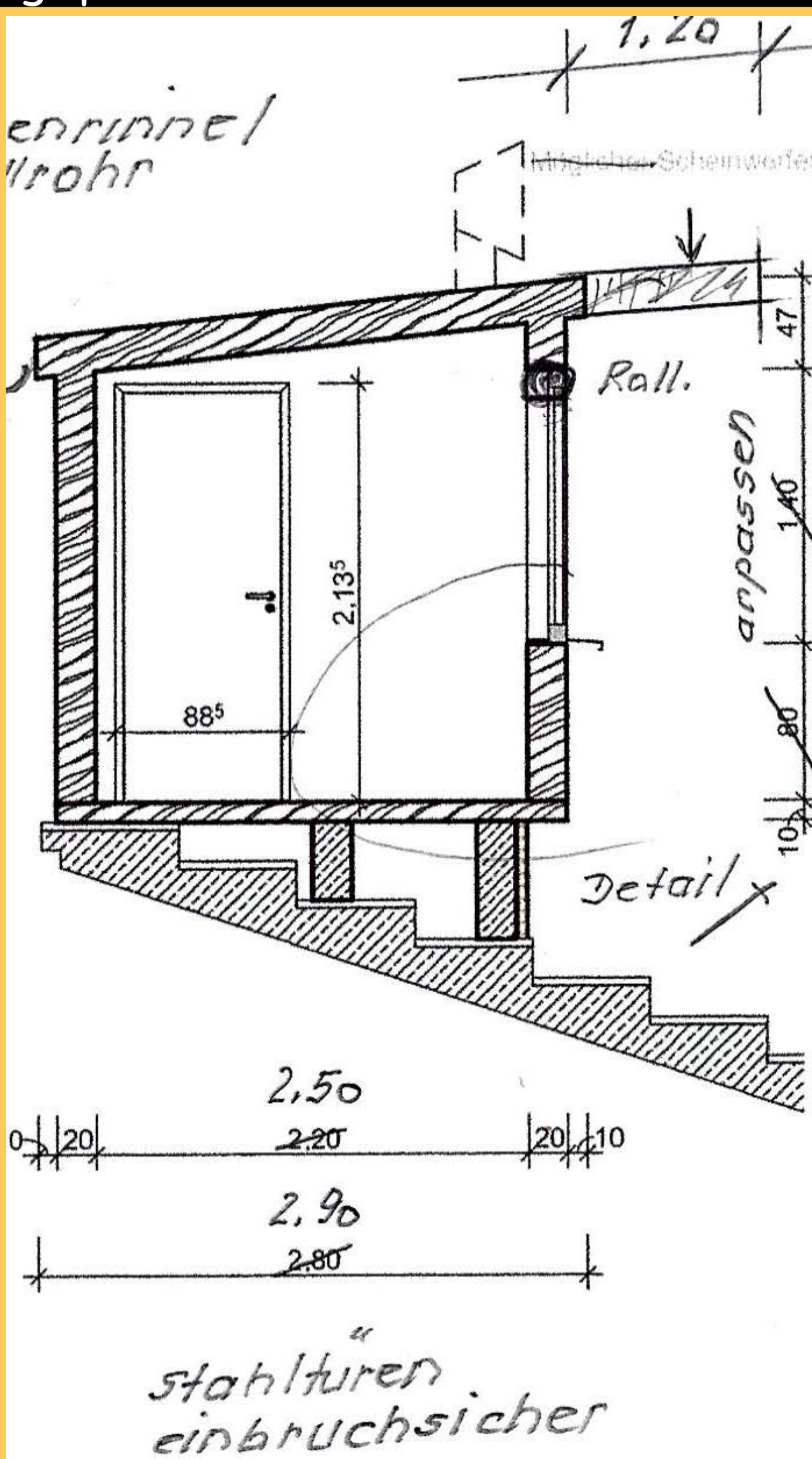
Von Dirk Fellendorf bereitgestellte Bauzeichnung für das neue FOH.
